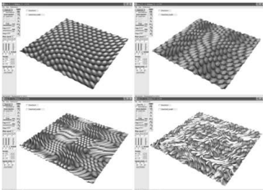
Рис. 9 – Варіанти розрахованої простої та складної асиметричної інтерпольованої перфорованої структури для підвищення енергетичного обміну в турбуленізованих середовищах
