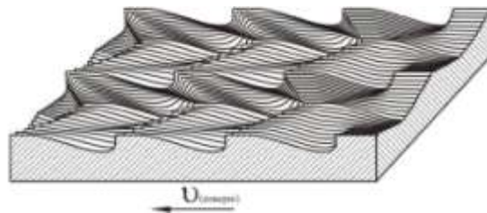
Рис. 5 – Варіант складної порції поверхні з урахуванням перетікання при заданій турбулізації потоку для збільшення енергообміну з середовищем
