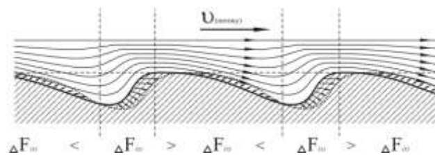
Рис. 2, а – Варіант інтерпольованого перерізу структур для роботи у більш енергетично-навантажених системах
