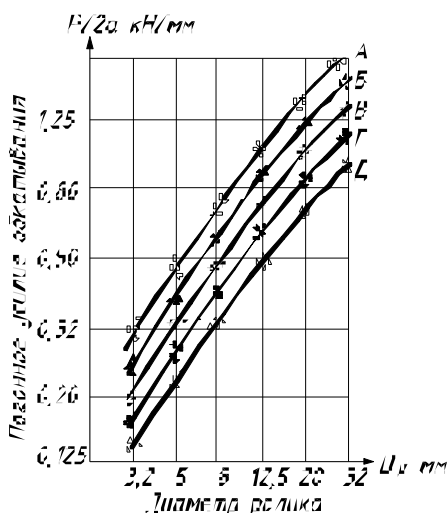
Рис. 4 – Зависимость погонного усилия обкатывания от диаметра ролика:
