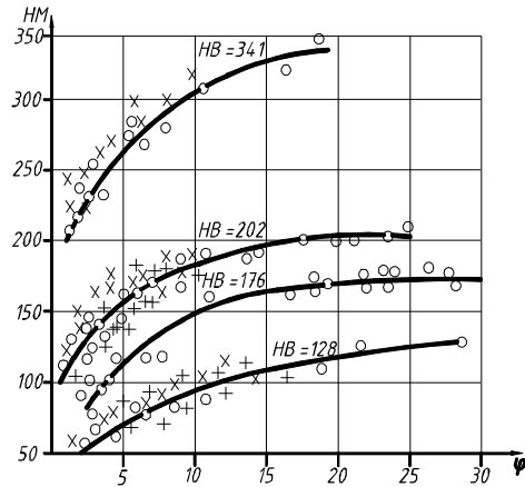
Рис. 2 – Зависимость среднего давления на отпечатке от среднего угла вдавливания: о – отпечатки шариков; х – отпечатки торообразных и бочкообразных роликов; + – отпечатки цилиндрических роликов
