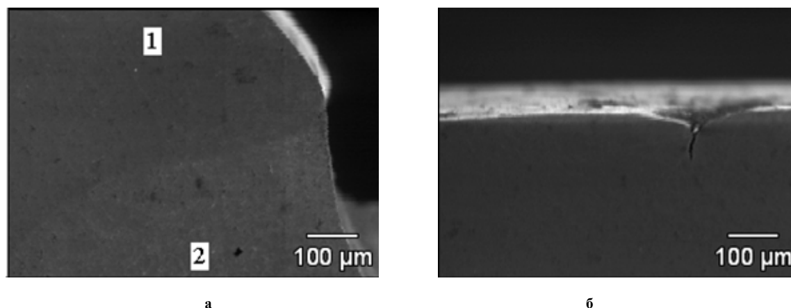
Рис. 9 – Мікроструктура (SEM) поверхні наплавлених шарів з використанням порошкового евтектичного електрода (а 1, б) і ванадій-хромового електрода (а 2)
