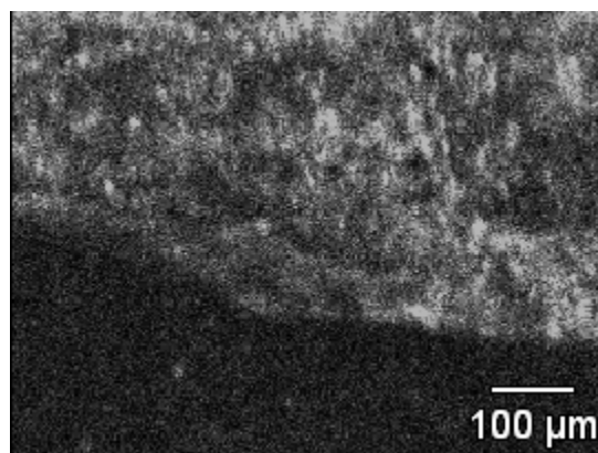
Рис. 10 – Розподіл атомів Si на поверхні тертя
