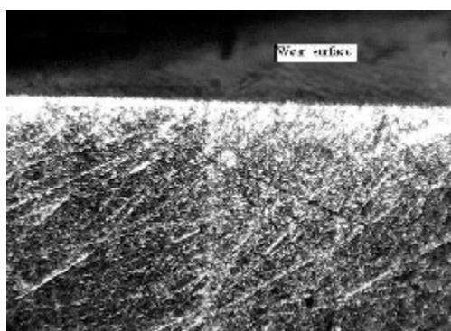
Рис. 8 – Мікроструктура покриття (x 200) наплавленого шару одержаного методом електродугового наплавлення з використанням евтектичного порошкового електроду системи Fe-Mn-C-B легovanого Si, Ni і Cr
