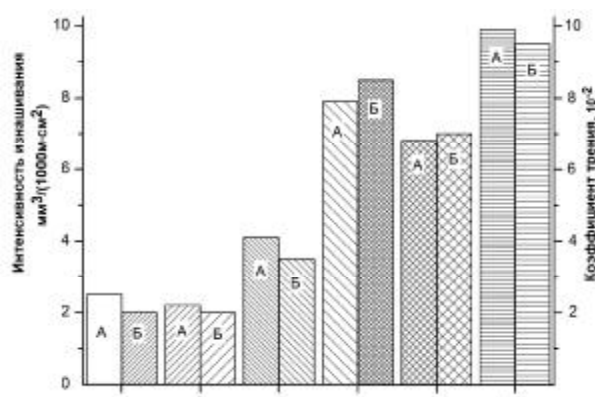
Рис.1 – Влияние материала контргтела на интенсивность изнашивания (А) и коэффициент трения (Б), ( P=20\text{МПа} , V=2,0\text{ м/с} ): 1,2,3 – аморфно-кристаллическое покрытие Zr-Al-B в парах трения с образцами БрОЦС6-6-3, АО-20, 30ХГСНА; 4,5,6 – покрытие из вольфрамсодержащего сплава типа BK-15 в парах трения с образцами БрОЦС6-6-3, АО-20, 30ХГСНА;
