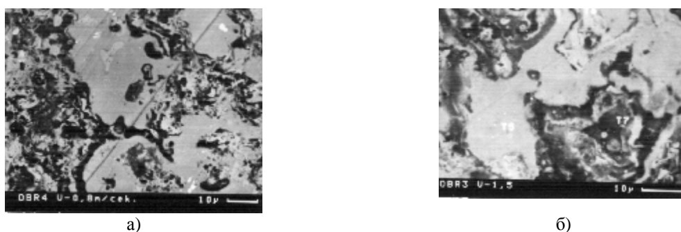
Рис.2 – Микрофотографии поверхностей трения аморфно-кристаллических покрытий в условиях граничного трения маслом МС-20 ( P=15\text{ МПа} ): а – при V=0,8\text{ м/с} ; б – при V=1,5\text{ м/с} ;
