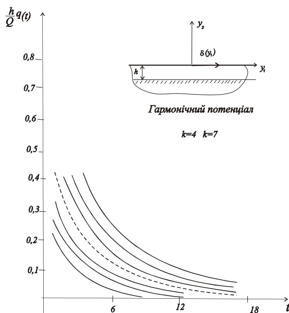
Рис. 2 – Контактна взаємодія під дією горизонтальної сили у випадку гармонічного потенціалу
