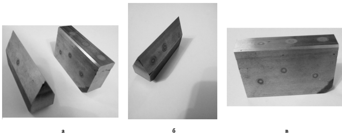
Рис. 3 – Робочі органи ножиць Н-32 з наплавленим покриттям. Робоча пара (а), ніж (б), упор (в)
