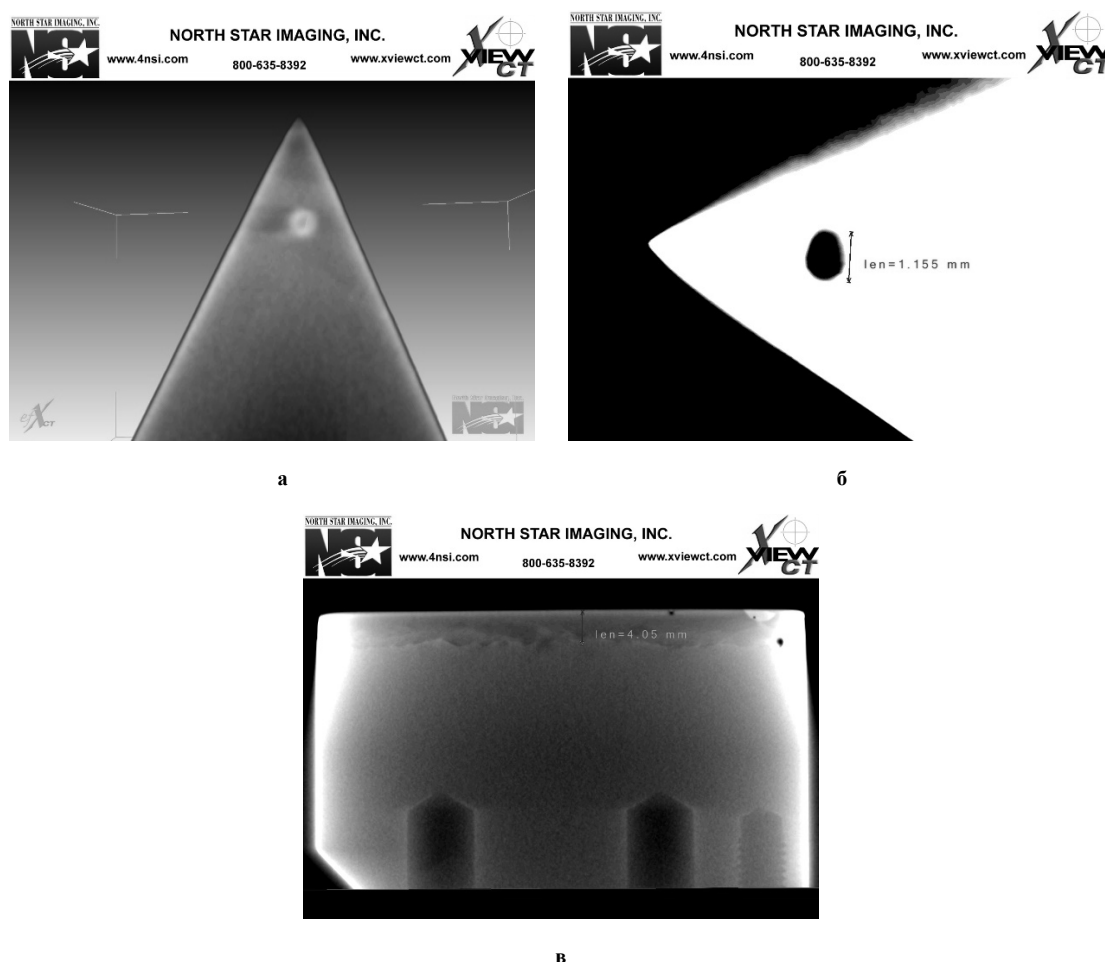
Рис. 4 – Томографія поверхні робочих органів ножиць Н-32 з захисним покриттям ніж (а, б), упор (в)
