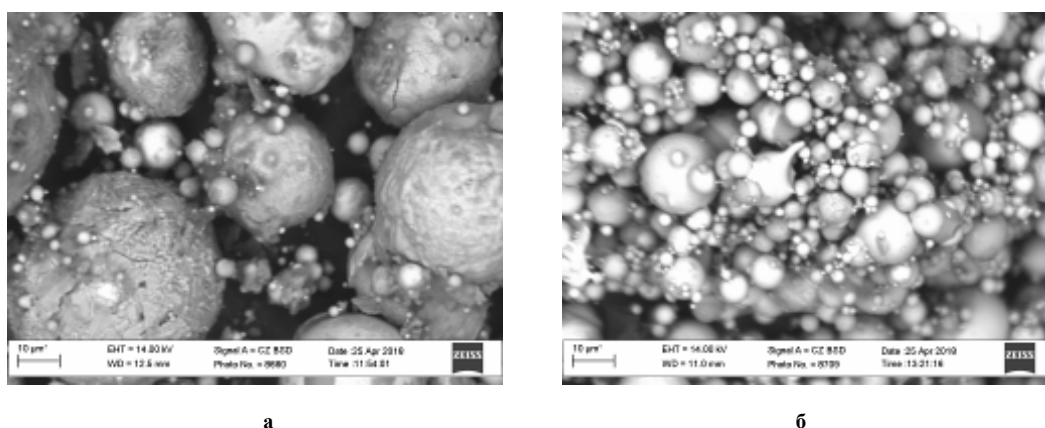
Рис. 7 – Розмір та форма краплин отриманих із ПД Х18Р3С2 залежно від тиску повітряного струменю: а – 0,6 МПа; б – 1,2 МПа
