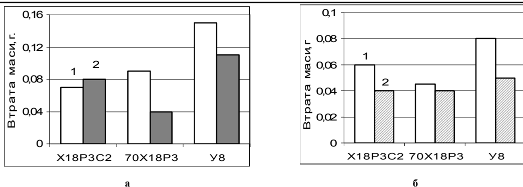
Рис. 12 – Зносостійкість покриттів із ПД: а – жорстко закріплені абразив; б – нежорстко закріплені абразив; 1 – 0,6 МПа; 2 – 1,2 МПа
