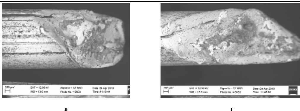
Рис. 6 – Торці дротів після наплення: а – У8, 0,6 МПа; б – У8, 1,2 МПа; в – ПД Х18Р3С2, 0,6 МПа; г – ПД Х18Р3С2, 1,2 МПа
