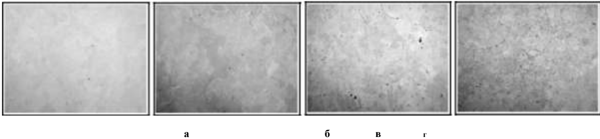
Рис. 8 – Выделение структурно-свободного цементита (500) в структуре бунтового проката диаметром 11,0 мм из стали С82D: а – скорость охлаждения 14 °С/с (класс В); б – скорость охлаждения 8 °С/с (класс С); в – скорость охлаждения 5,5 °С/с (класс D); г – скорость охлаждения 4,5 °С/с (класс Е)
