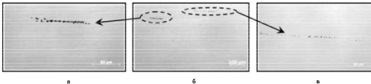
Рис. 6 – Допустимые неметаллические включения в бунтовом прокате из стали С78D диаметром 7,0 мм по ГОСТ 1778-70 (продольный шлиф): а – силикаты хрупкие (1 балл); б – общий вид неметаллических включений; в – оксиды строчечные (2 балл)
