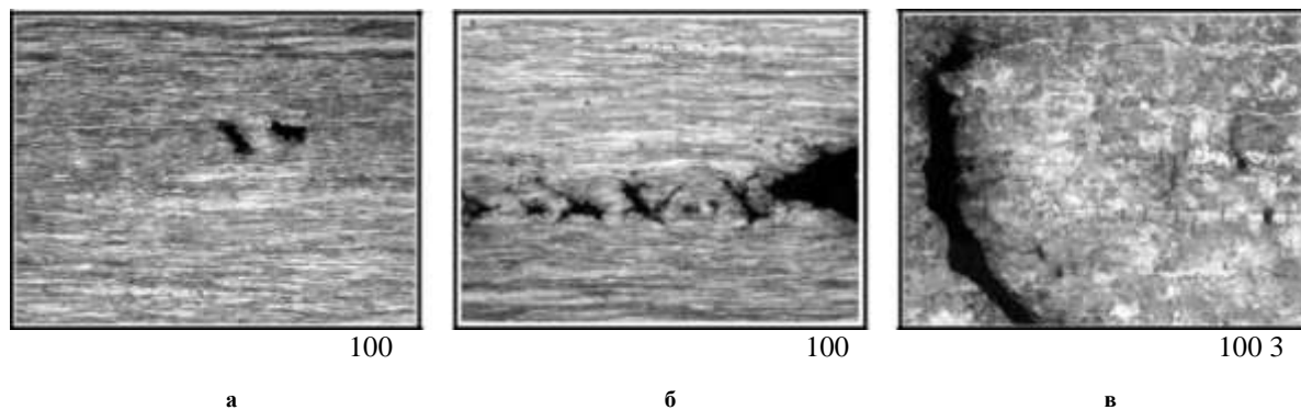
Рис. 3 – Необратимое повреждение бунтового проката, вызывающее преждевременное разрушение холоднотермомеханической проволоки диаметром 7,2 мм из стали S82D (V 0,072 %): а – осевая часть проката вблизи зоны ликвационной полосчатости; б – V-образная трещина вблизи мартенсита; в – развитие микротрещины вблизи участков перлита 5 балла (по ГОСТ 8233-56)
