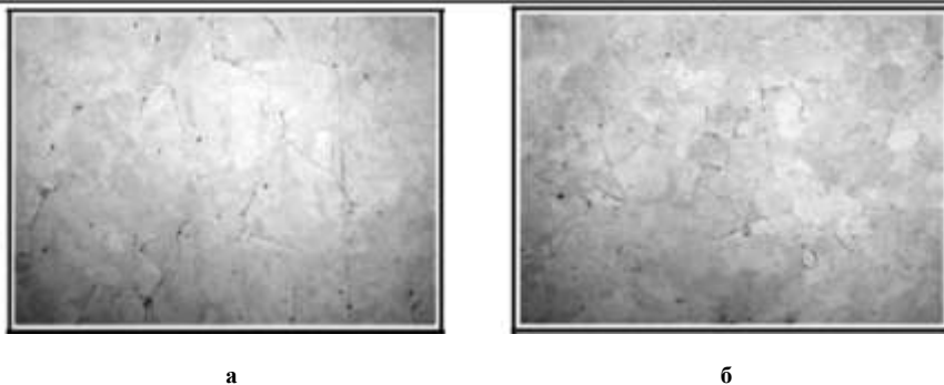
Рис. 4 – Структурно свободный цементит ( 500) по границам перлитных зерен в бунтовом прокате из стали С82D диаметром 11,0 мм (содержание хрома 0,27 %): а – скорость охлаждения 7 °C/c; б – скорость охлаждения 5,8 °C/c
