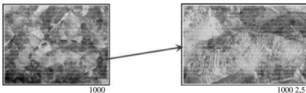
Рис. 5 – Неравномерность формирования перлитной структуры в бунтовом прокате из стали марки С72D диаметром 6,5 мм (количество сорбитообразного перлита менее 35 %)
