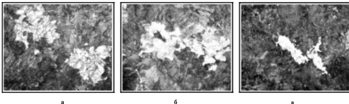
Рис. 2 – Мартенсит в осевой зоне (1000) бунтового проката из стали S82D диаметром 12,0 мм (продольный шлиф): а – содержание хрома 0,25 %; б – содержание ванадия 0,068 %; в – без легирующих элементов
