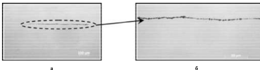
Рис. 7 – Недопустимые неметаллические включения в бунтовом прокате из стали С72D диаметром 6,5 мм по ГОСТ 1778-70 (продольный шлиф): а – общий вид неметаллического включения; б – силикаты хрупкие (4 балл)
